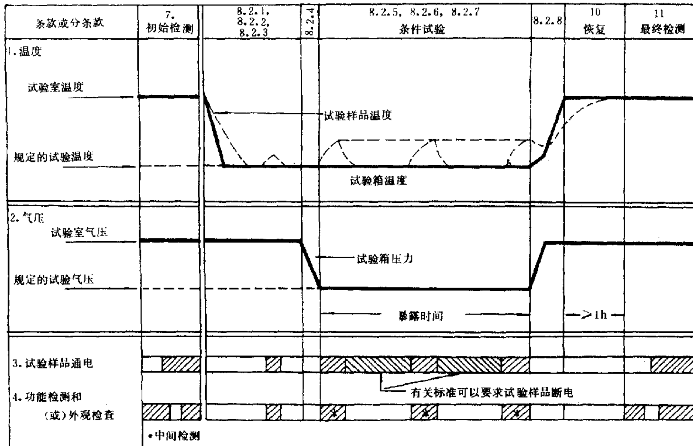
图 2 散热试验样品的试验剖面图
