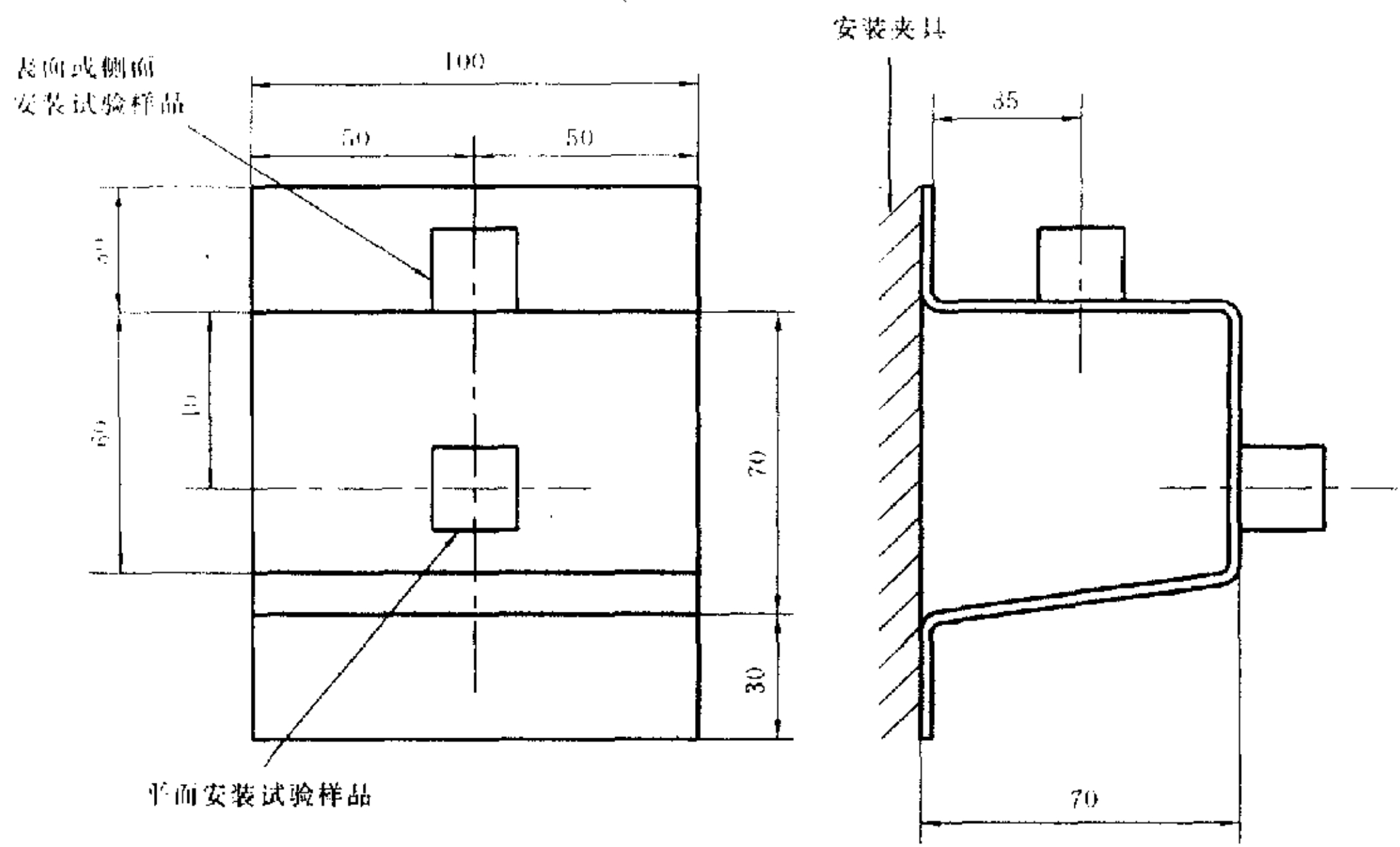
图 5 灯座的安装
