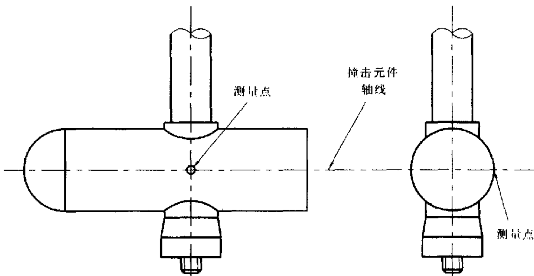
图 6 测量点的获取
