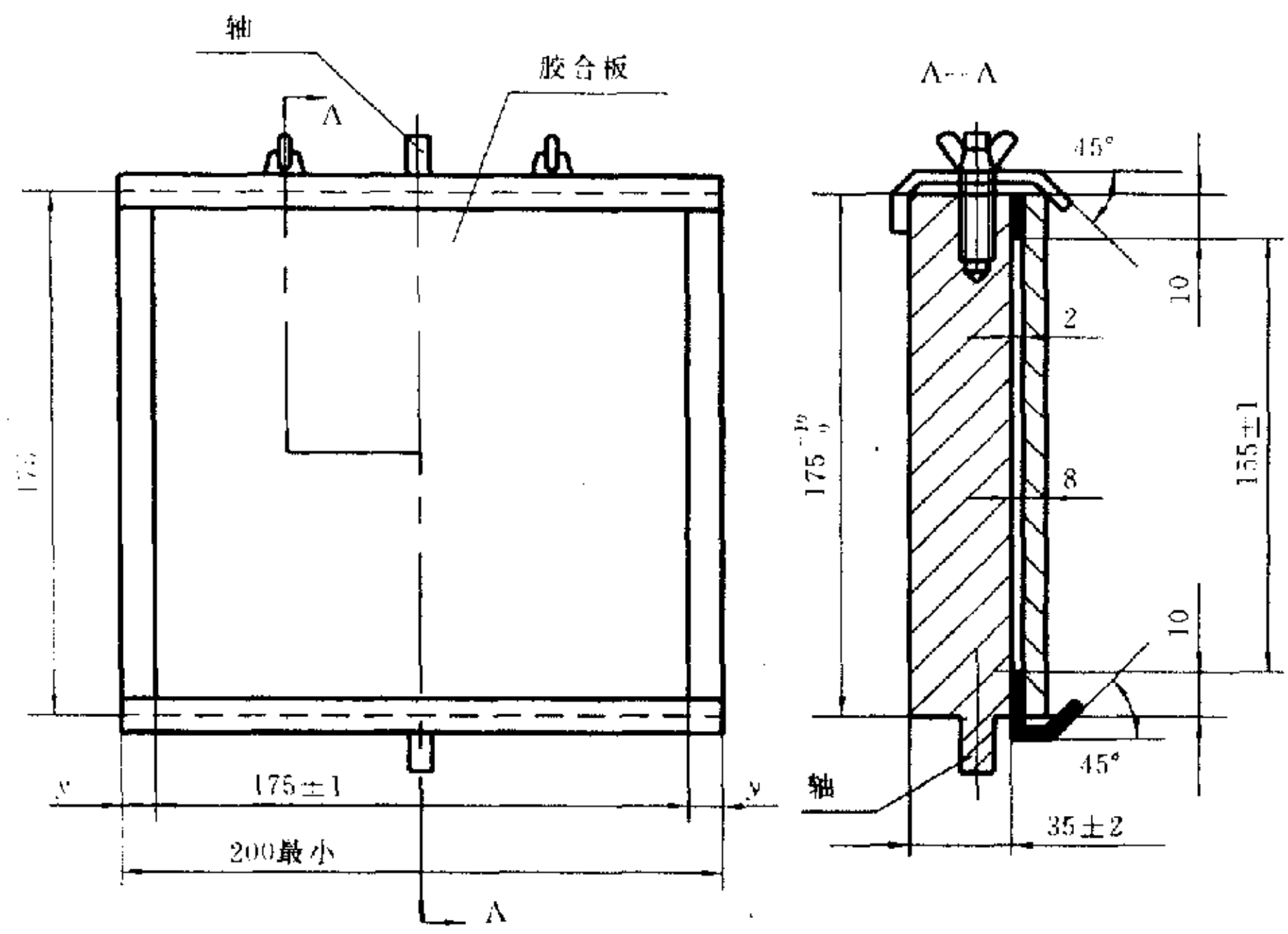
图3 安装夹具
