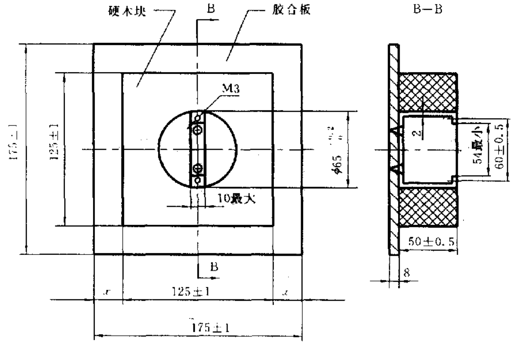
图4 平面型开关的安装
