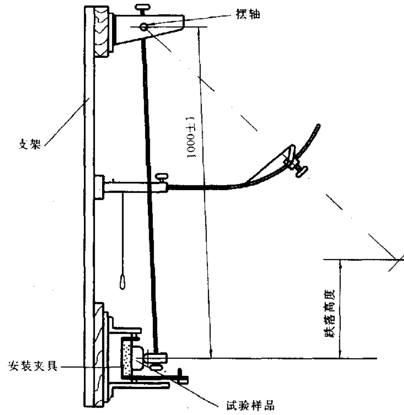
图1 试验装置
