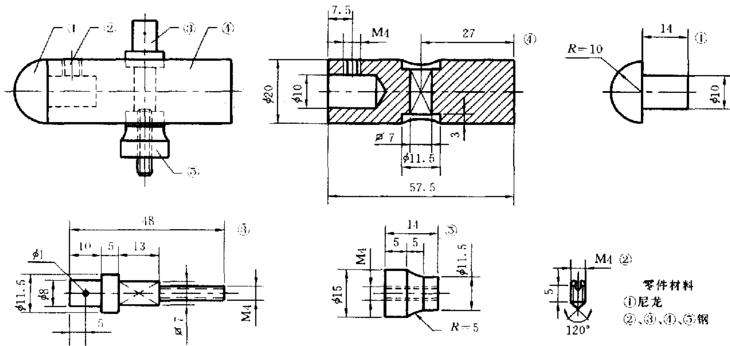
图2 撞击元件
